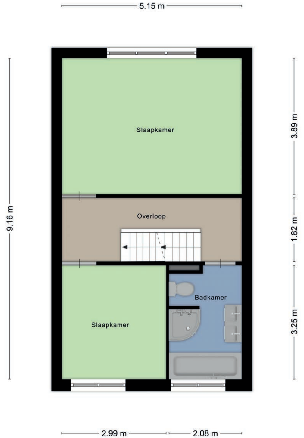
TWEEDE VERDIEPING
