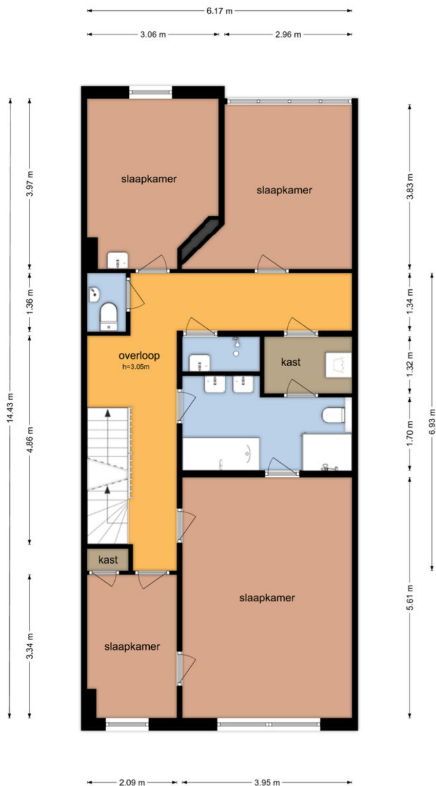
Willem de Zwijgerstraat 1 - Utrecht Eerste Verdieping
