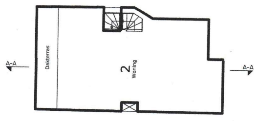
1e verdieping 1:100
