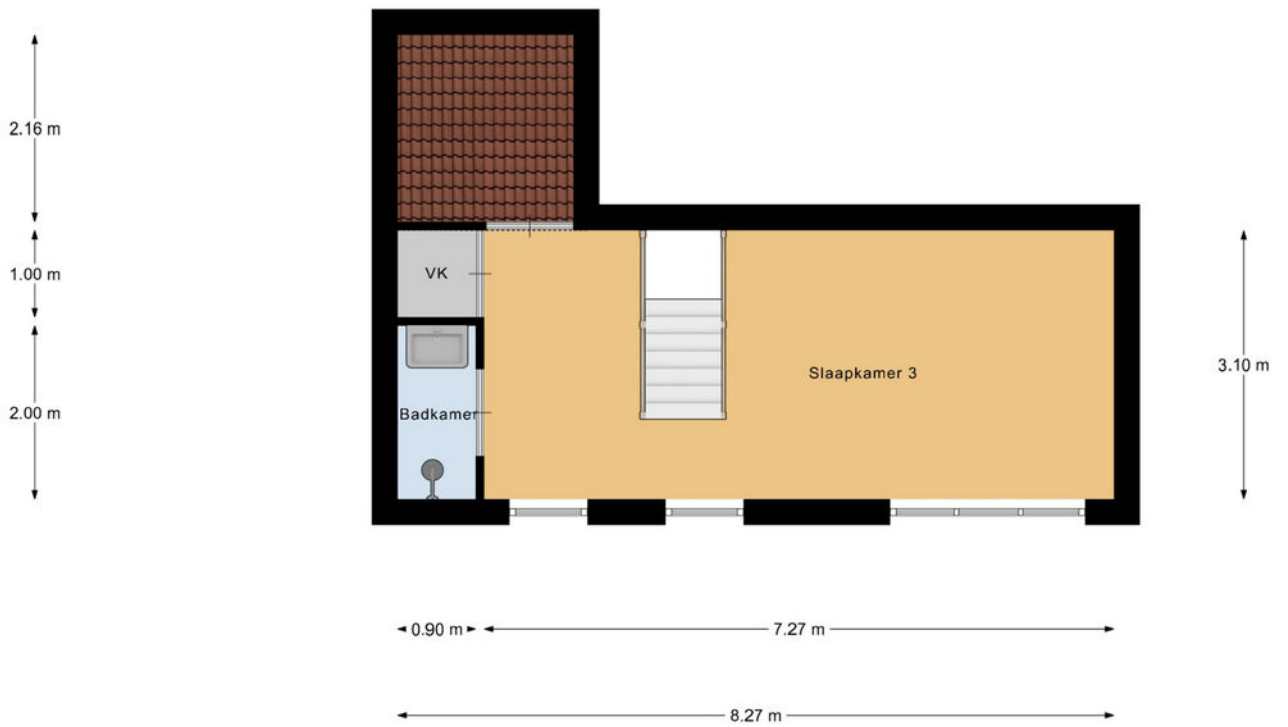
2e Verdieping
