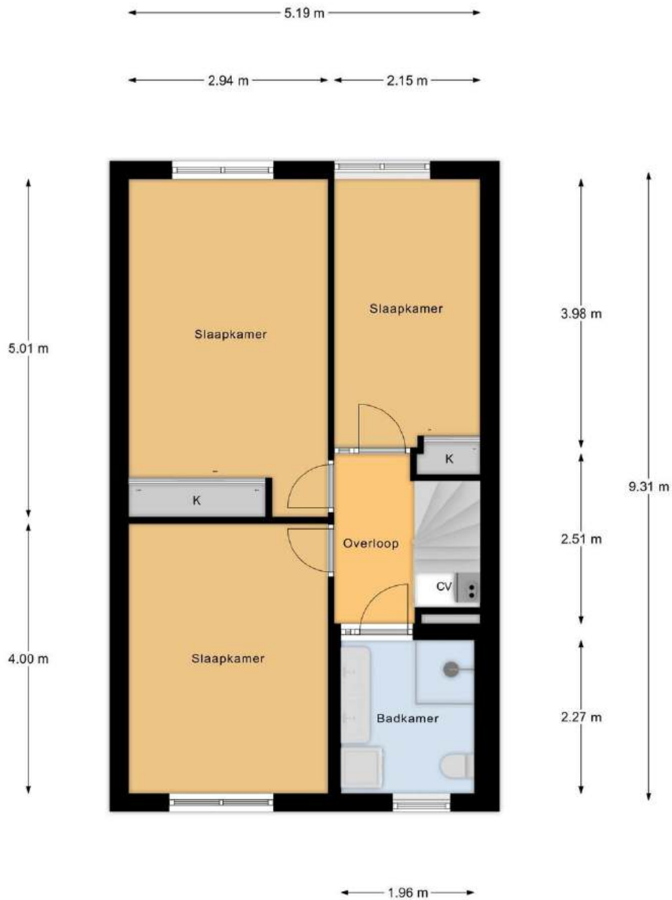
1e Verdieping
