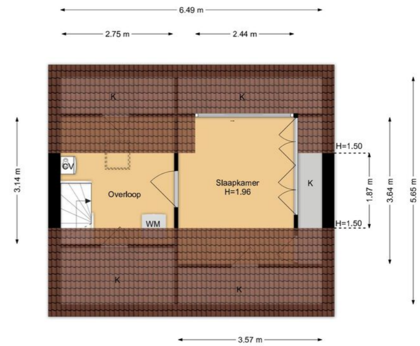
2e Verdieping Emmaweg 6, Zandvoort R.M. Vastgoedpresentatie| Aan deze plattegrond kunnen geen rechten worden ontleend
