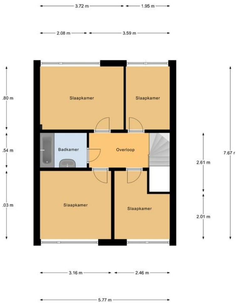
1e Verdieping
