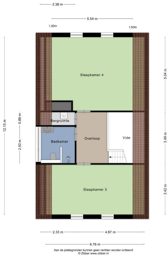
Der Grundriss der Etage mit ungefähren Maßen.
