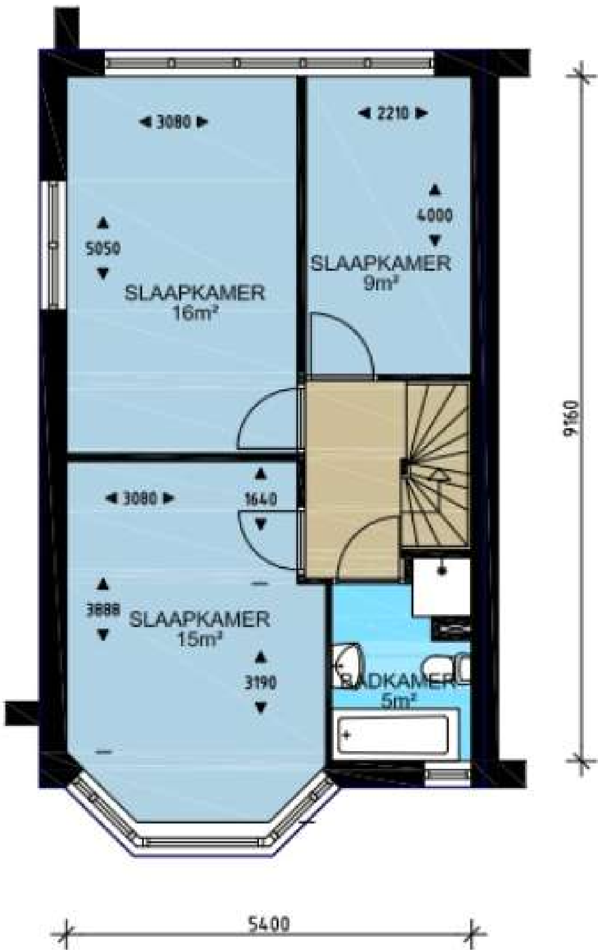
1e verdieping
