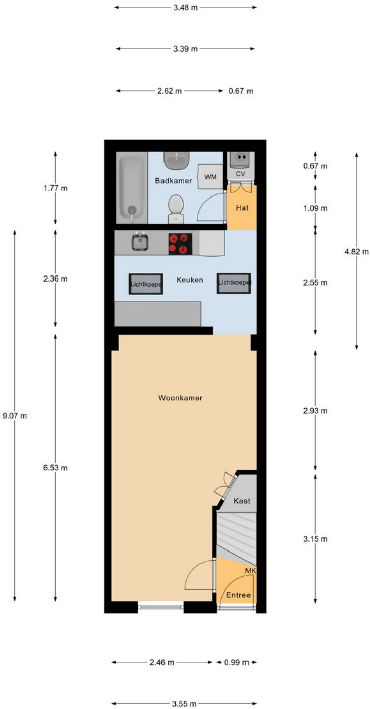
Begane Grond
