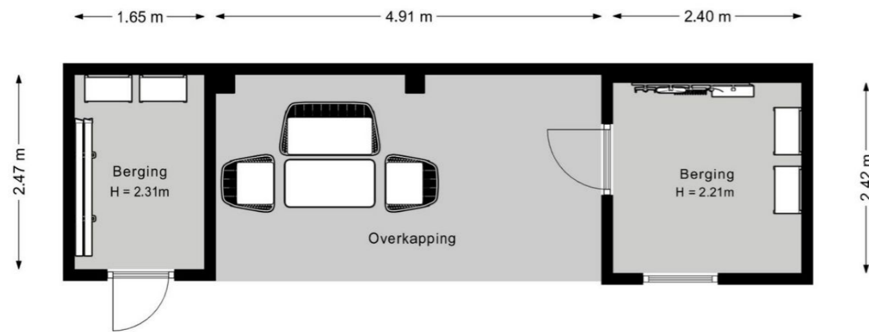
Plattegrond berging Aan deze tekening kunnen geen rechten worden ontleend
