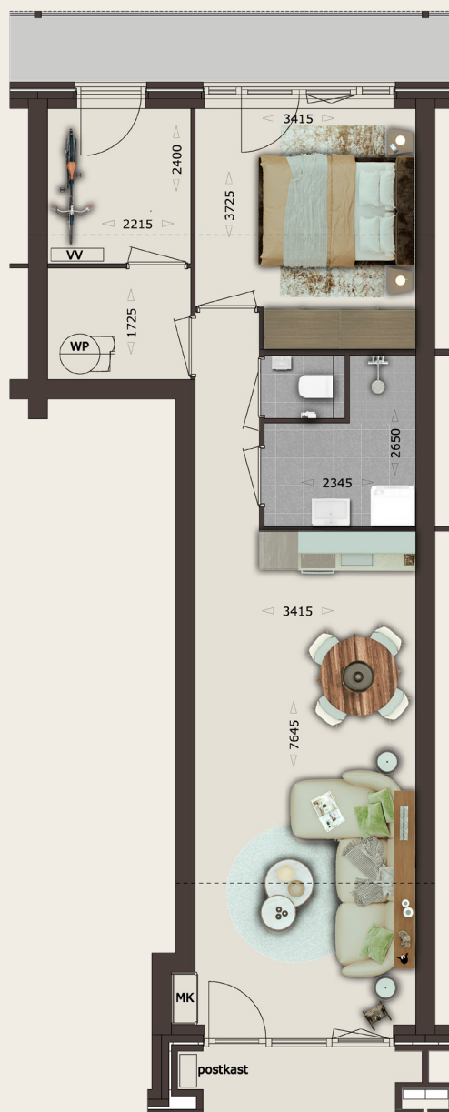
Begane grond
