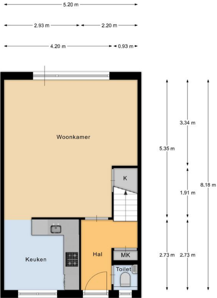
Begane grond
