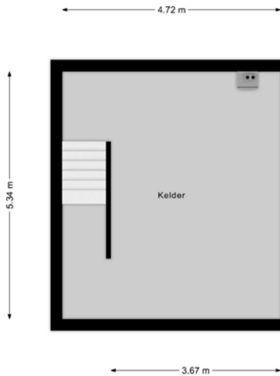
Indeling kelder
