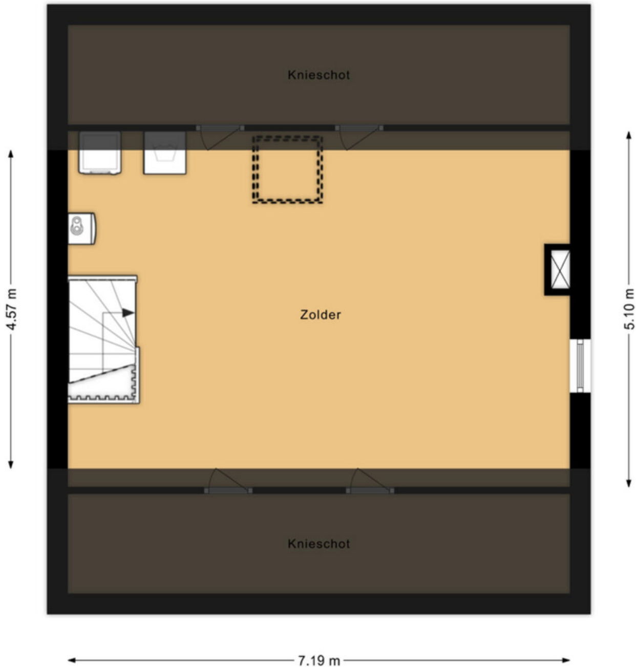
Tweede verdieping Klein Doesburg 32 Heerde
