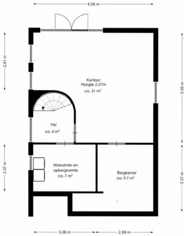
woonruimte 1 tuinniveau
