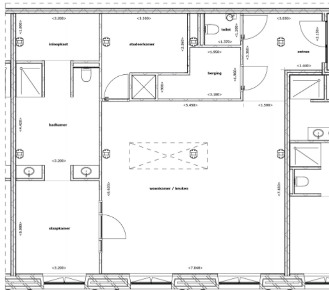
Plattegrond verdieping 01 1:50
