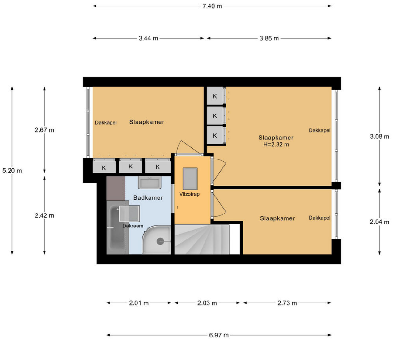
1e Verdieping
