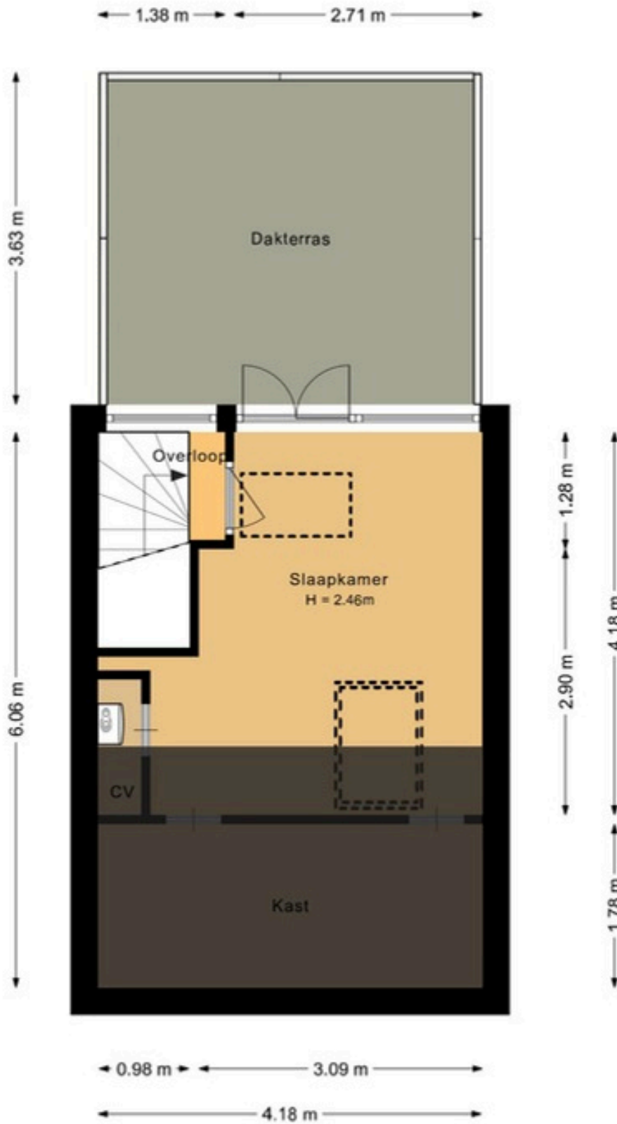
Tigrisstraat 23 Tweede verdieping
