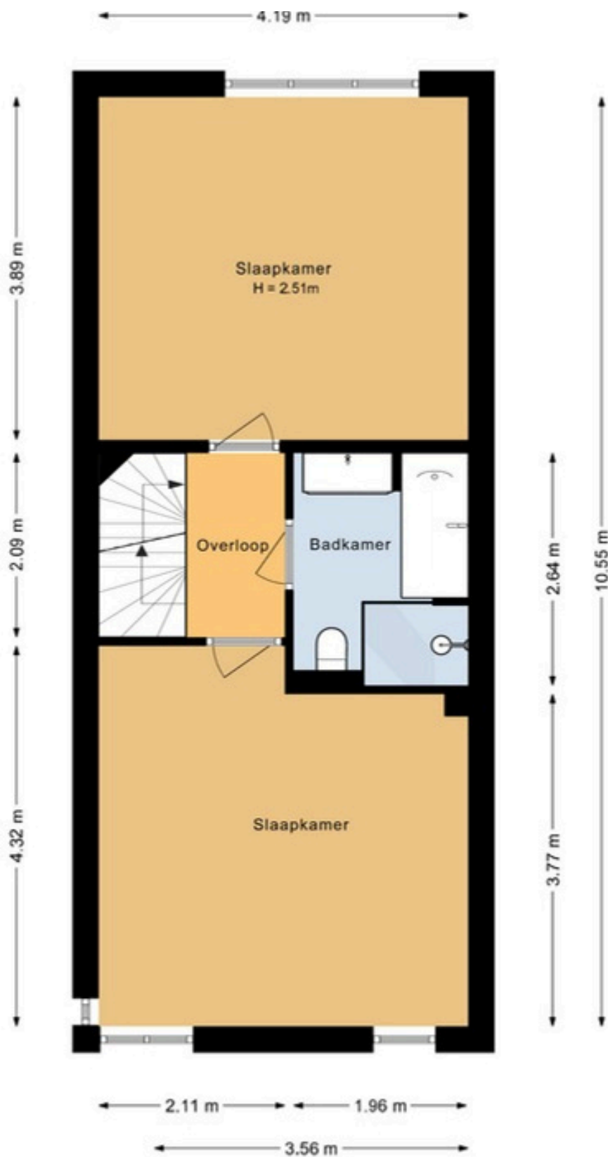
Tigrisstraat 23 Eerste verdieping
