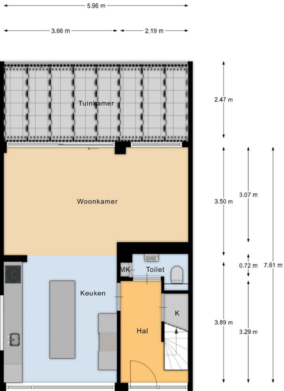
Begane grond
