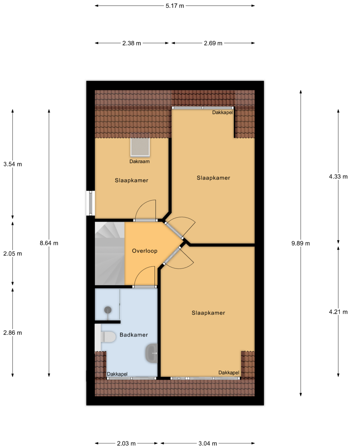
1e Verdieping
