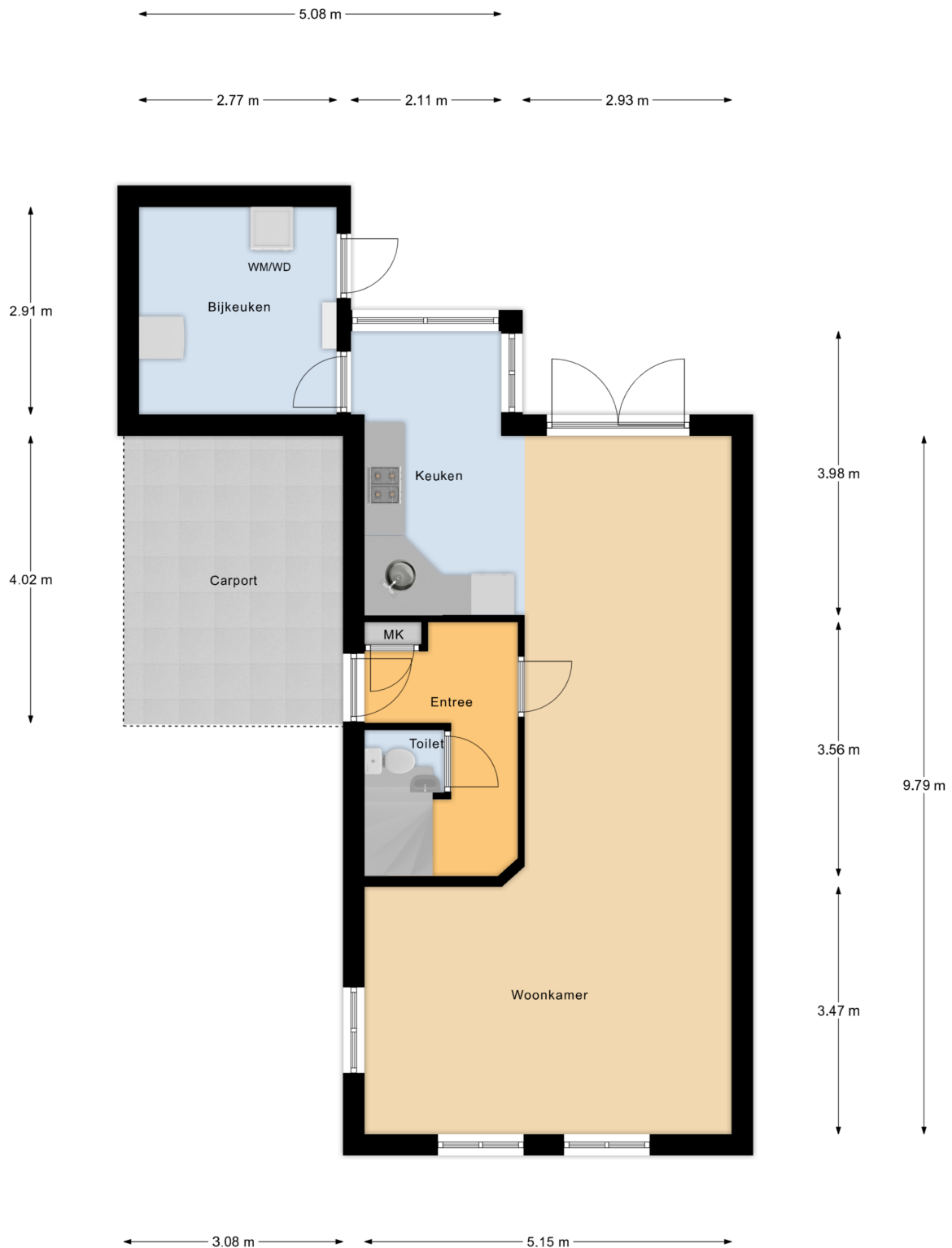
Begane Grond
