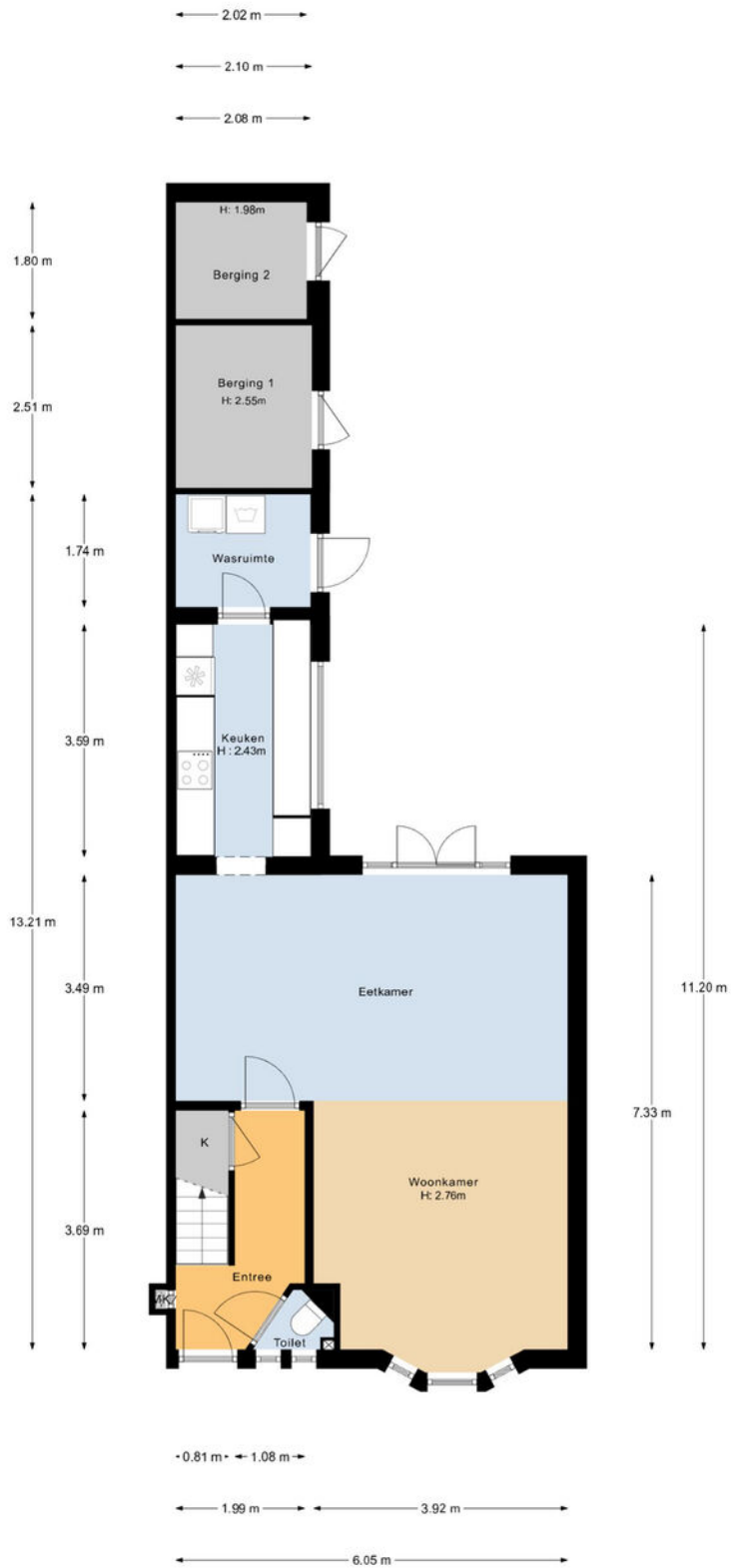
Begane grond
