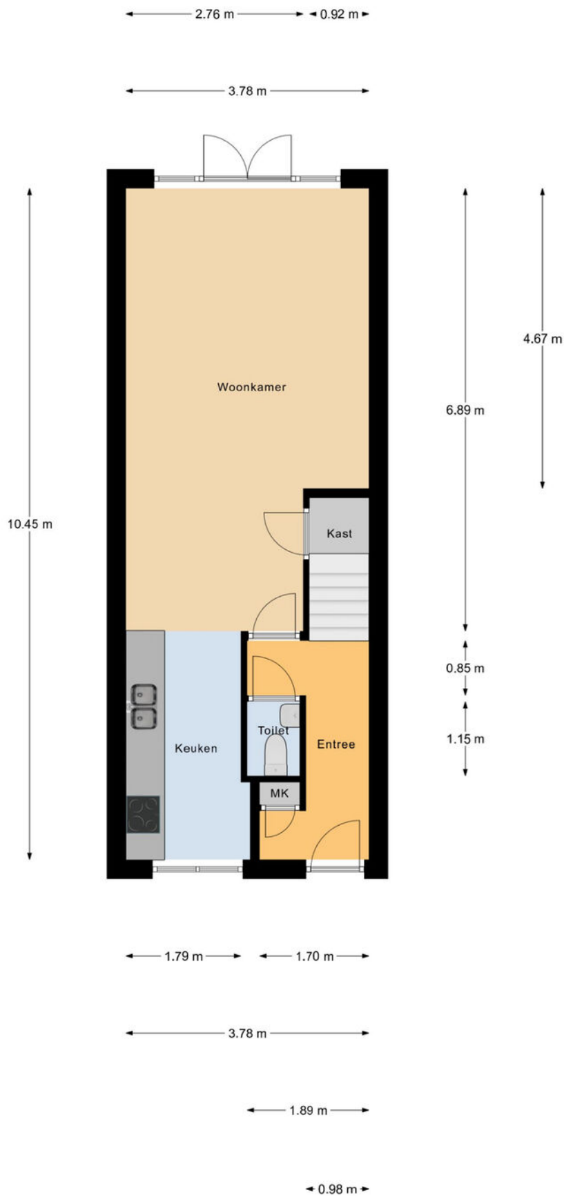
Begane Grond
