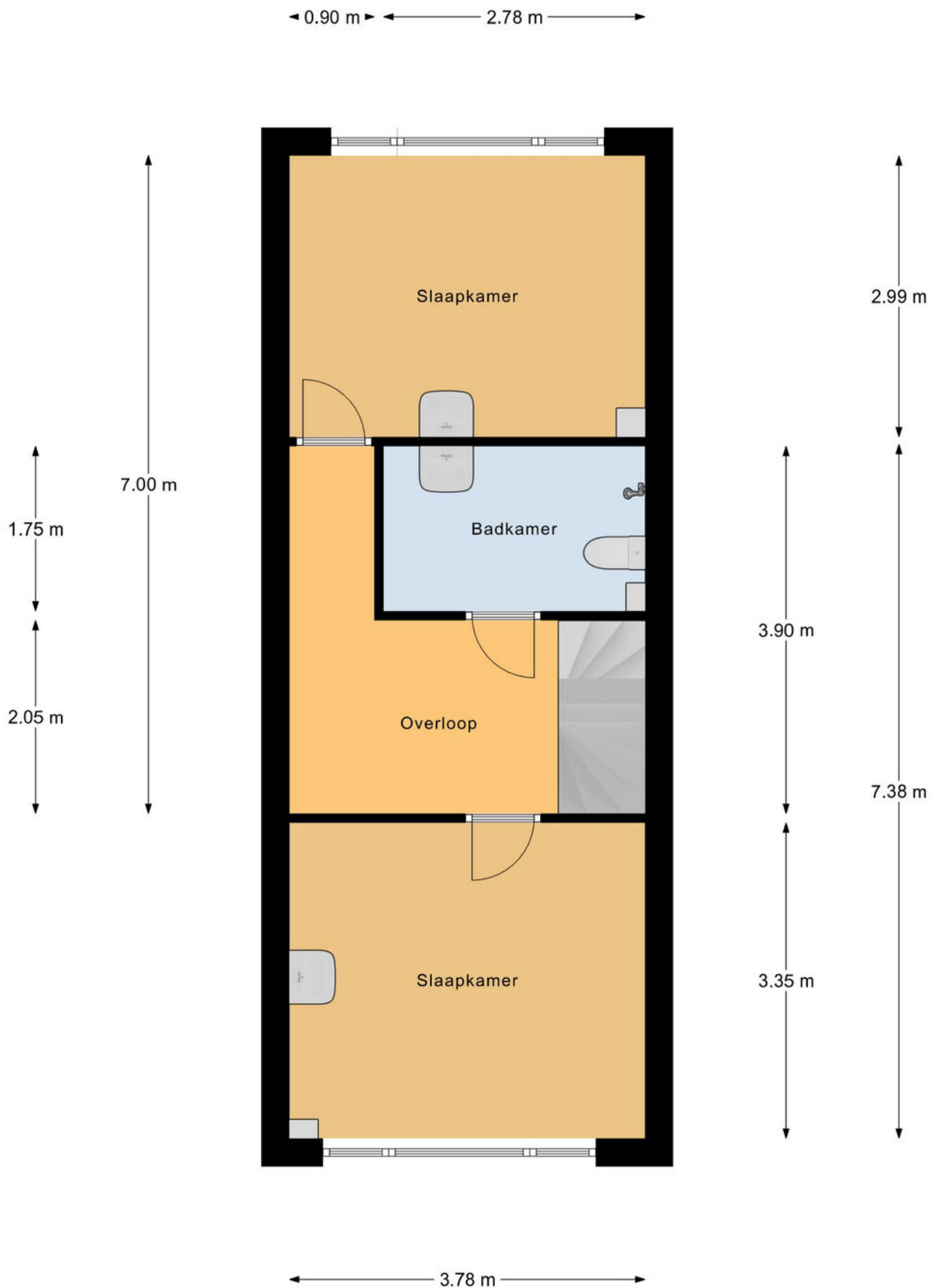
1e Verdieping
