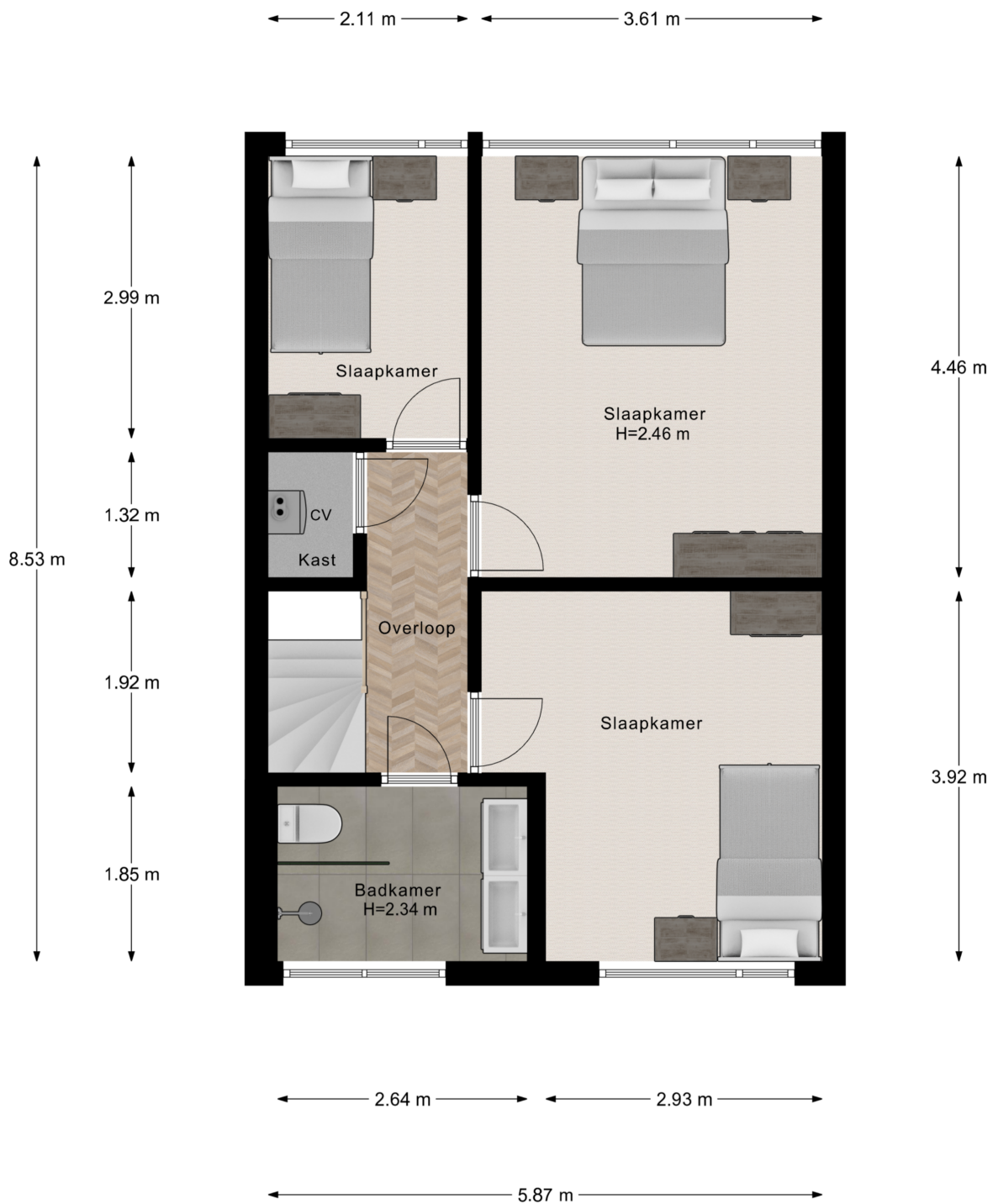
2e Verdieping
