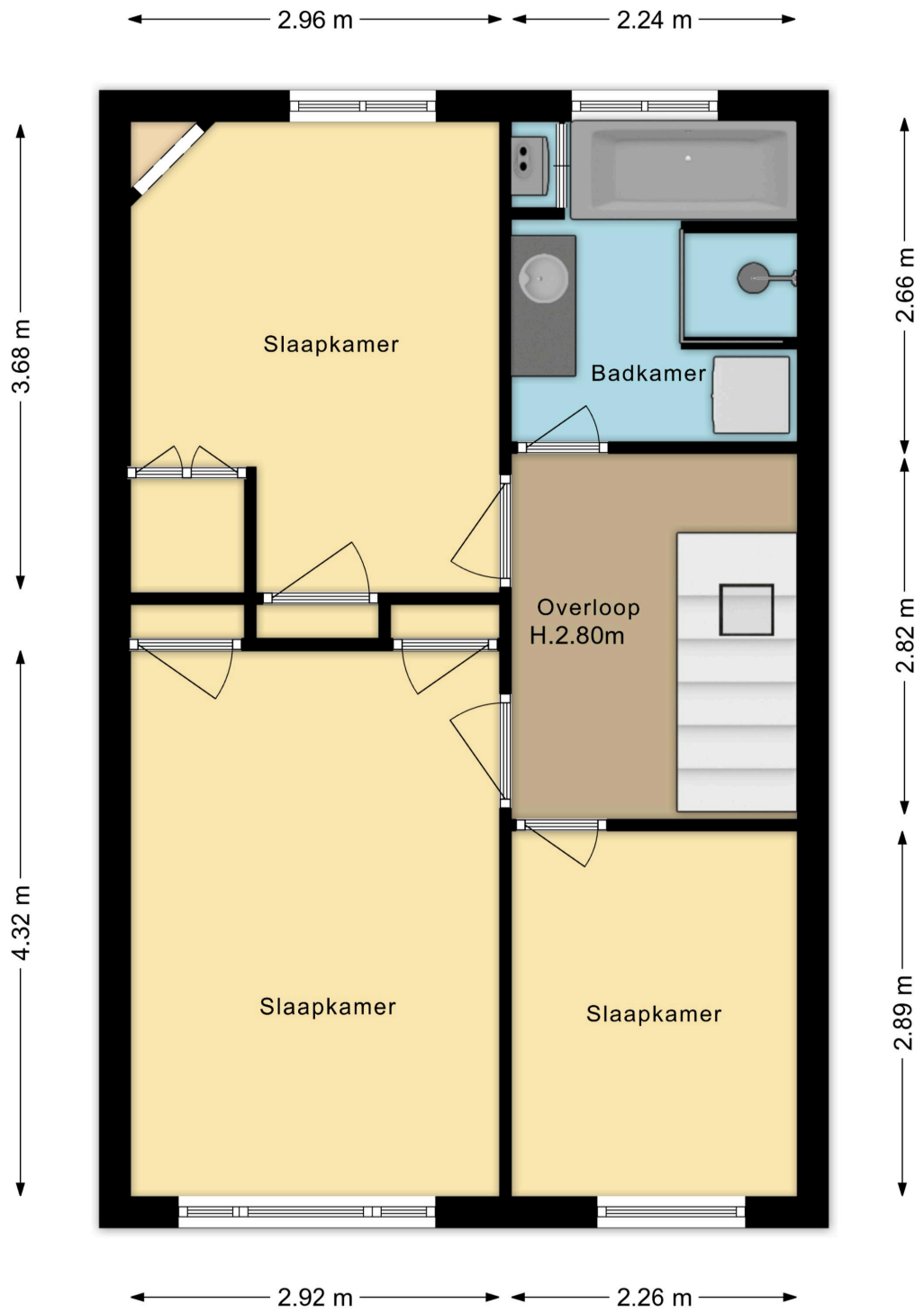
Verdieping Pieter Maritzstraat 9
