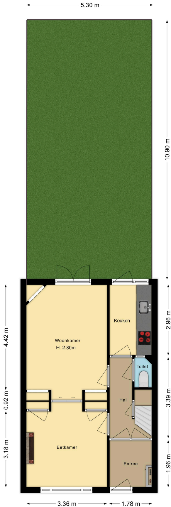
Begane grond met perceel Pieter Maritzstraat 9
