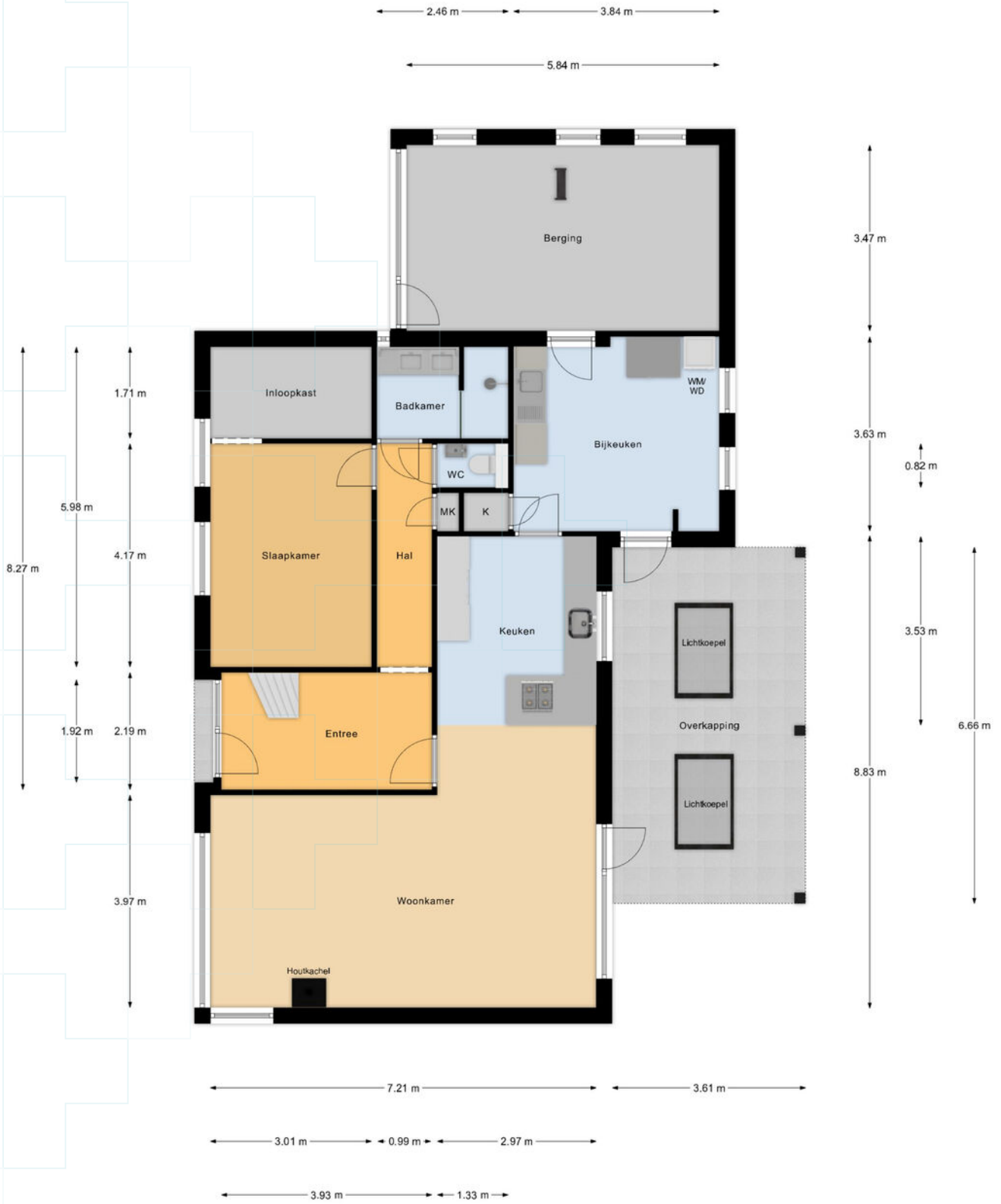
Begane Grond
