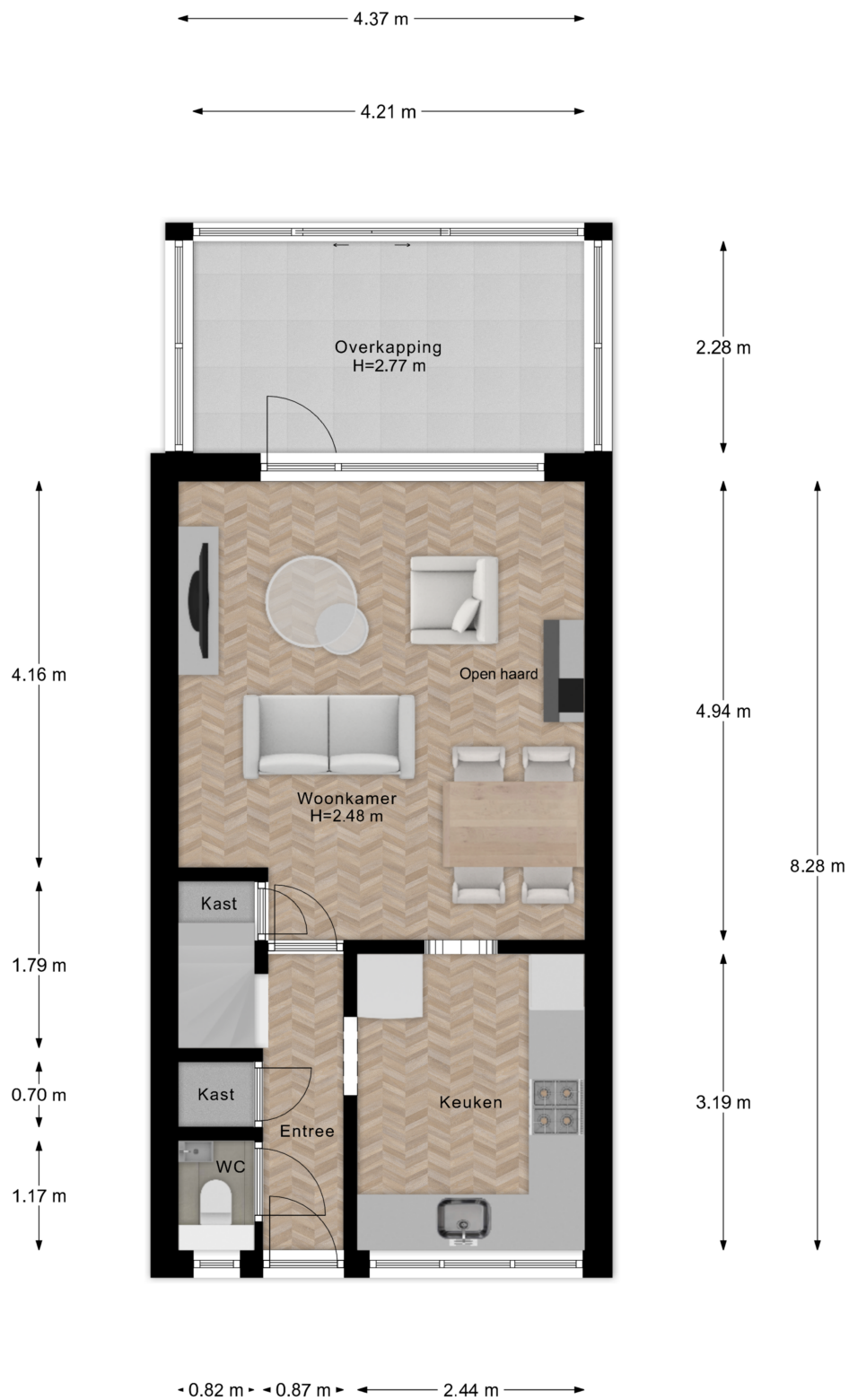
Begane Grond
