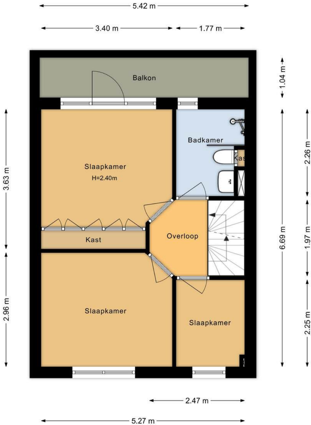
Eerste verdieping Abraham Kuiperstraat 6 Heemstede
