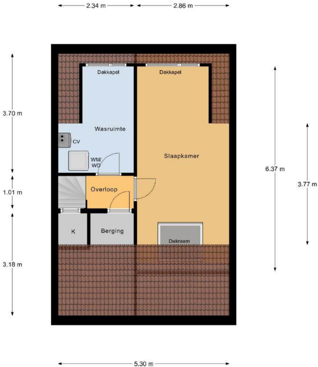
2e Verdieping
