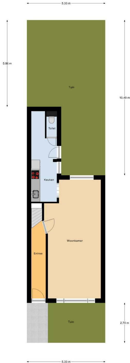
Begane Grond Tuin
