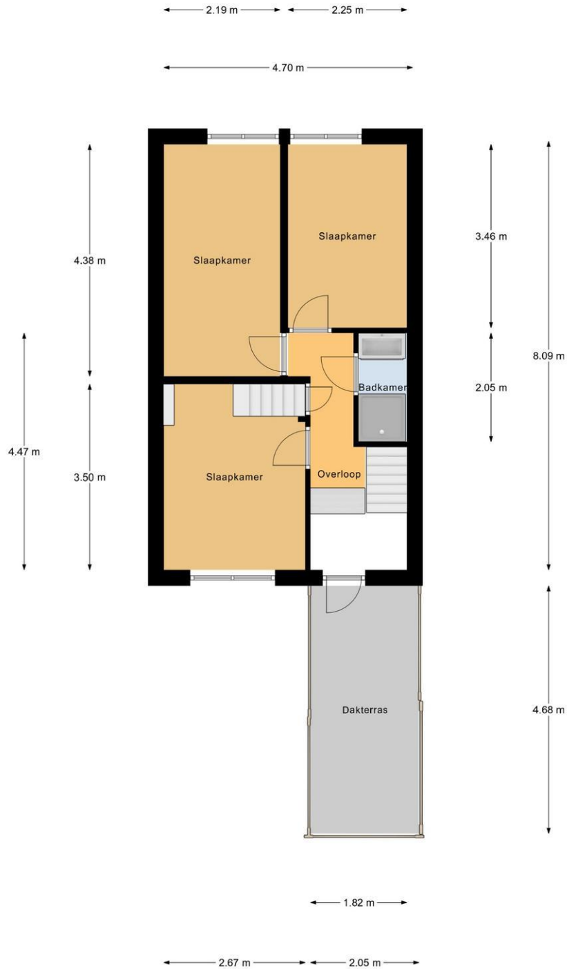
1e Verdieping
