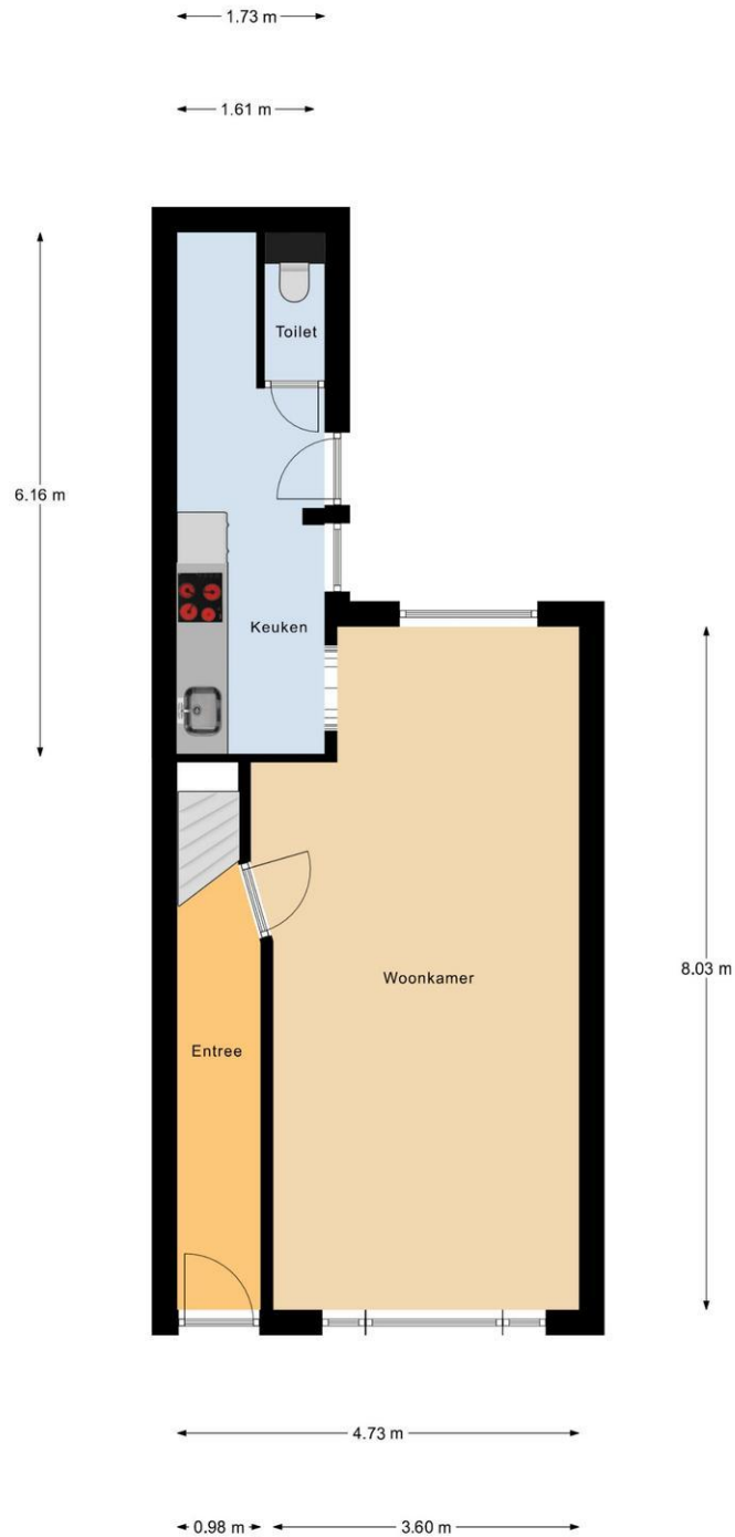
Begane Grond
