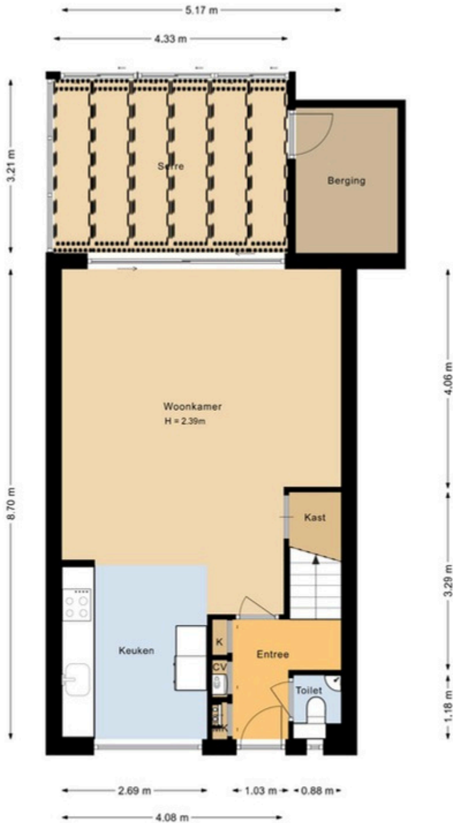
Graanstraat 37 Purmerend Begane Grond
