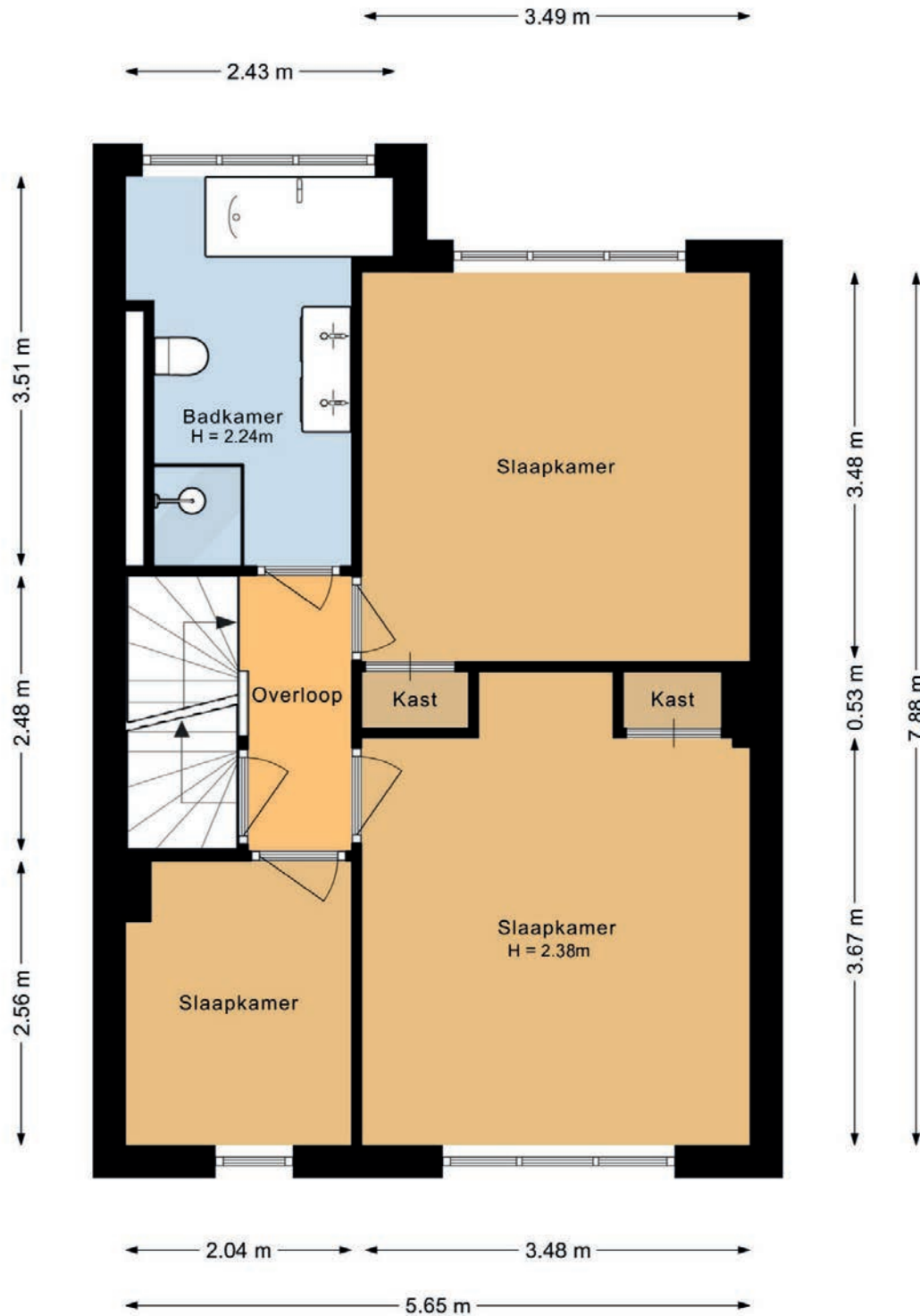
EERSTE VERDIEPING
