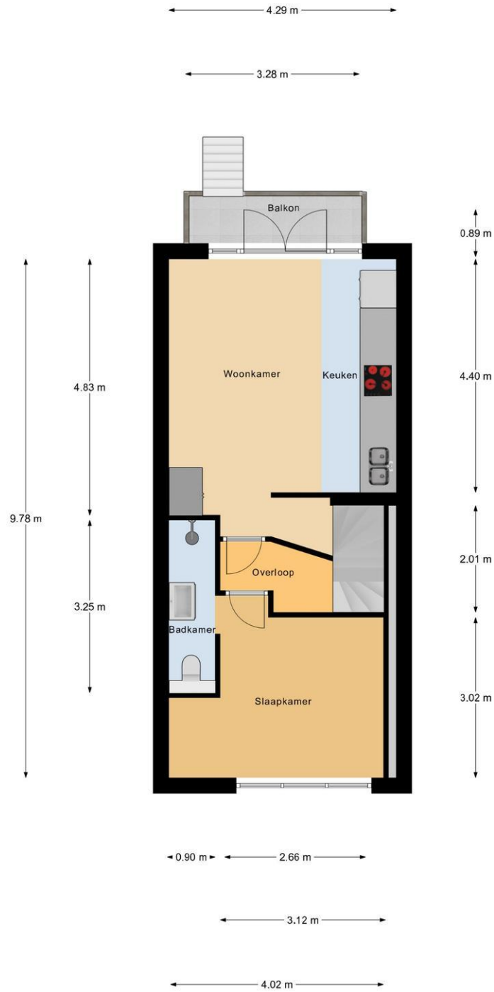
1e Verdieping
