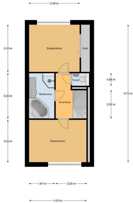
2e Verdieping
