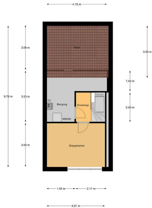
3e Verdieping
