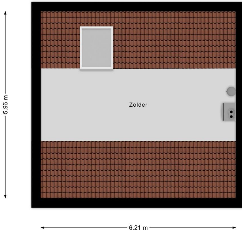
Tweede verdieping
