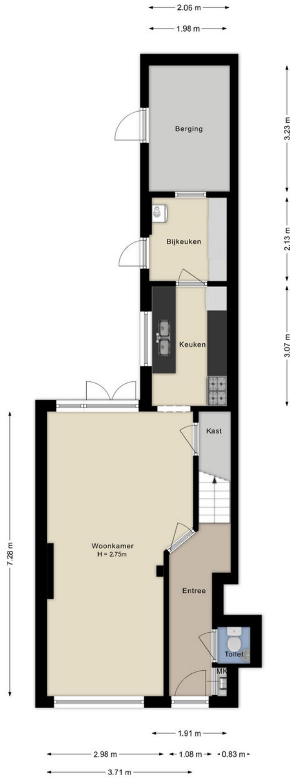
Begane grond Van Rijckevorsel van Kessellaan 70, 's-Hertogenbosch Aan de plattegronden kunnen geen rechten worden ontleend
