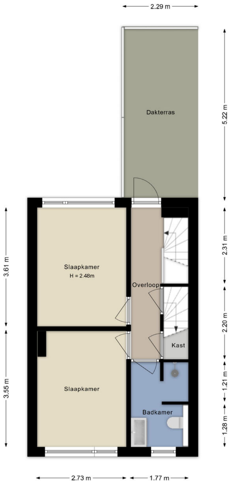
Eerste verdieping Van Rijkevorsel van Kessellaan 70, 's-Hertogenbosch
