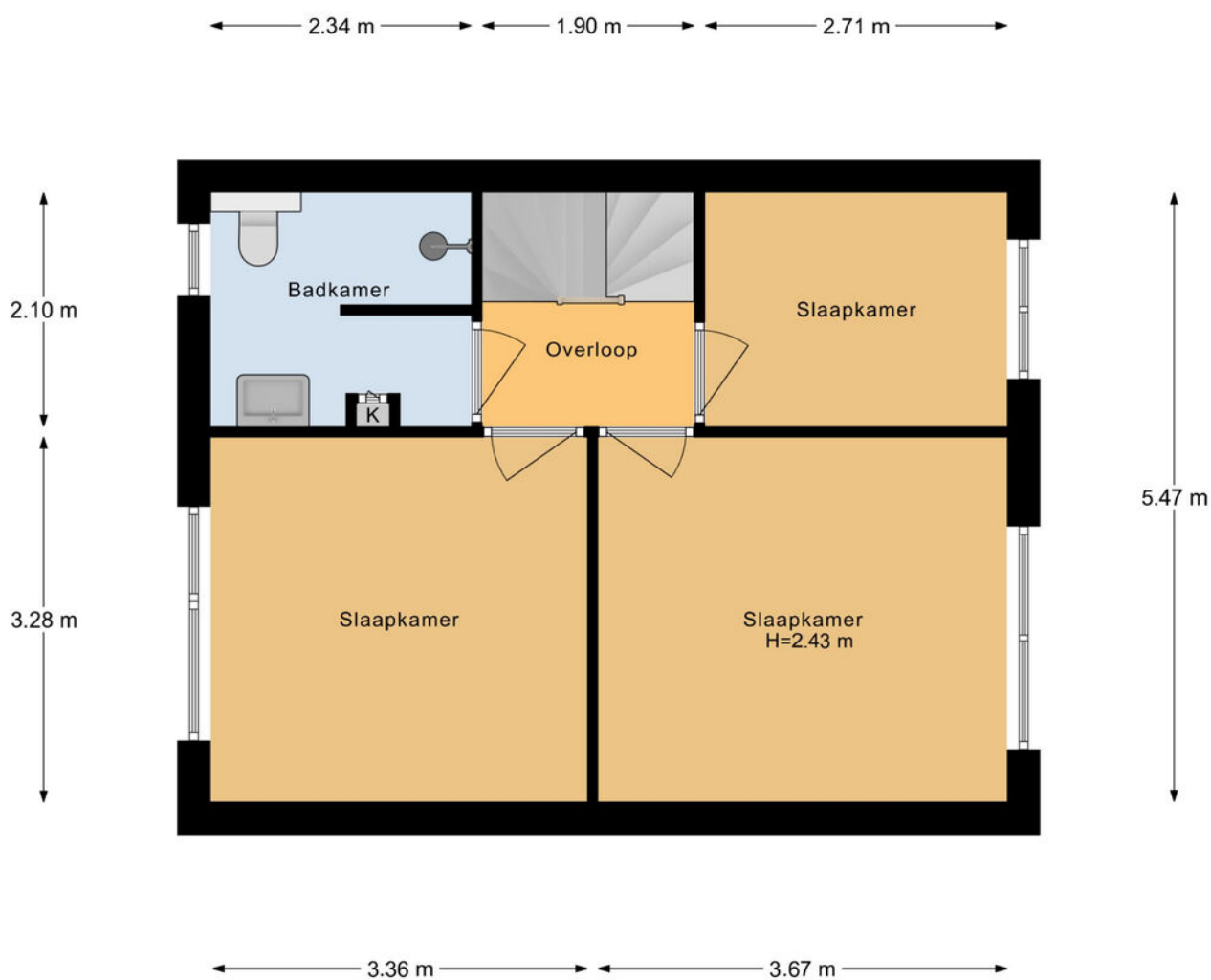
1e Verdieping
