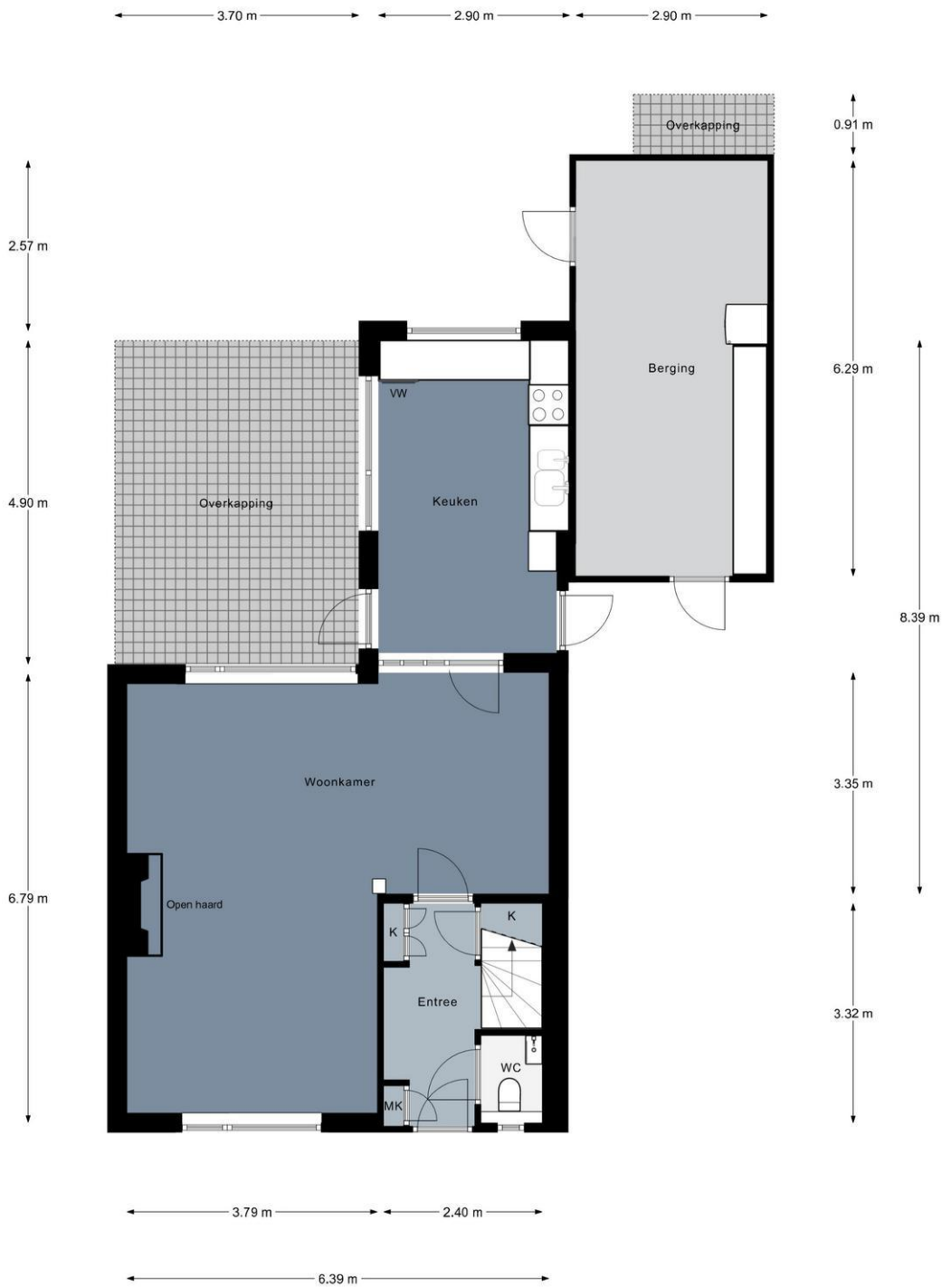
Begane Grond
