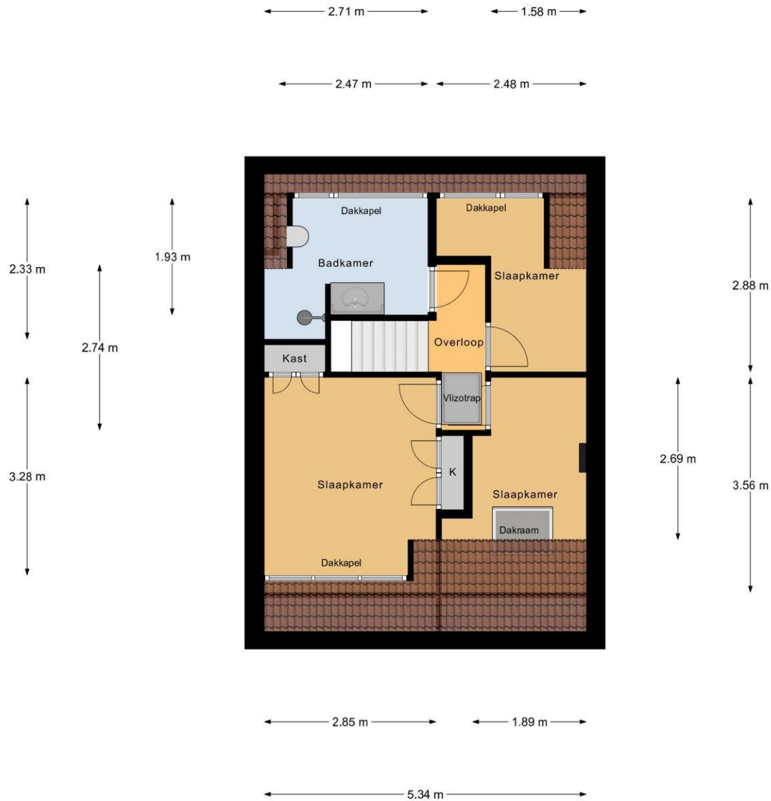
1e Verdieping
