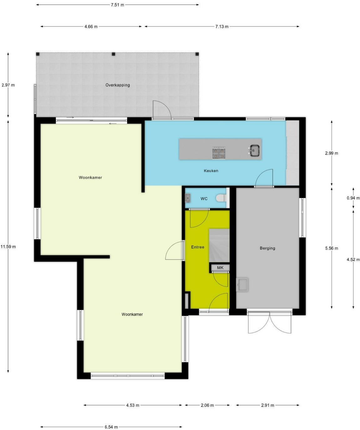
Begane Grond
