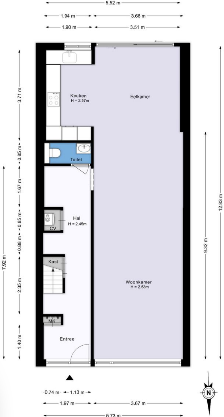
Bevelandsezijweg 12 - Amstelveen Begane grond
