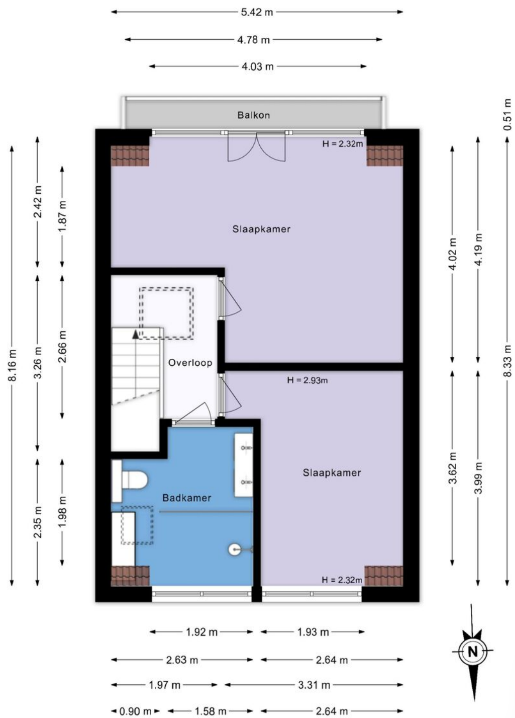
Bevelandsezijweg 12 - Amstelveen Tweede verdieping
