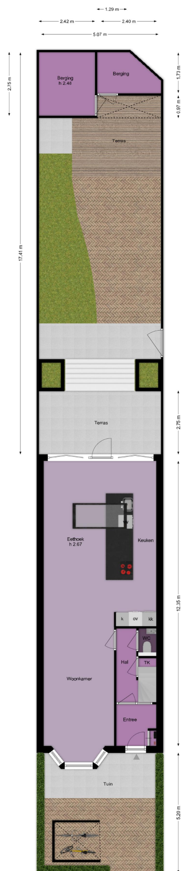
SITUATIE ZWARTEWEG 47 BENNEBROEK Aan de maatvoering kunnen geen rechten worden ontleend.
