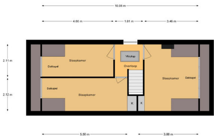
3e Verdieping
