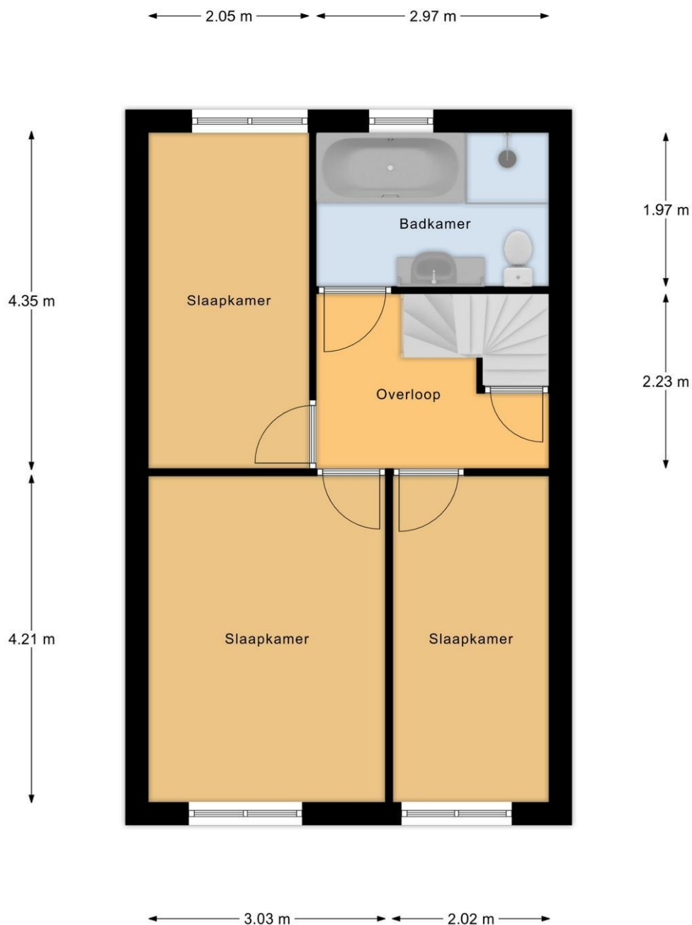
1e Verdieping
