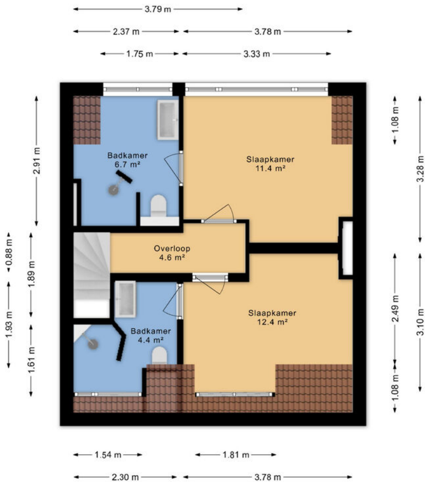
Burgemeester Engelbertsstraat 66 Zandvoort 2e Verdieping
