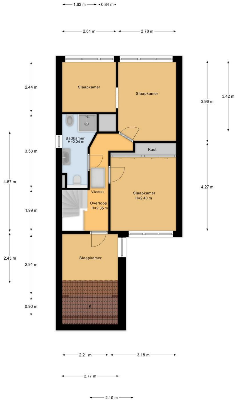
1e Verdieping
