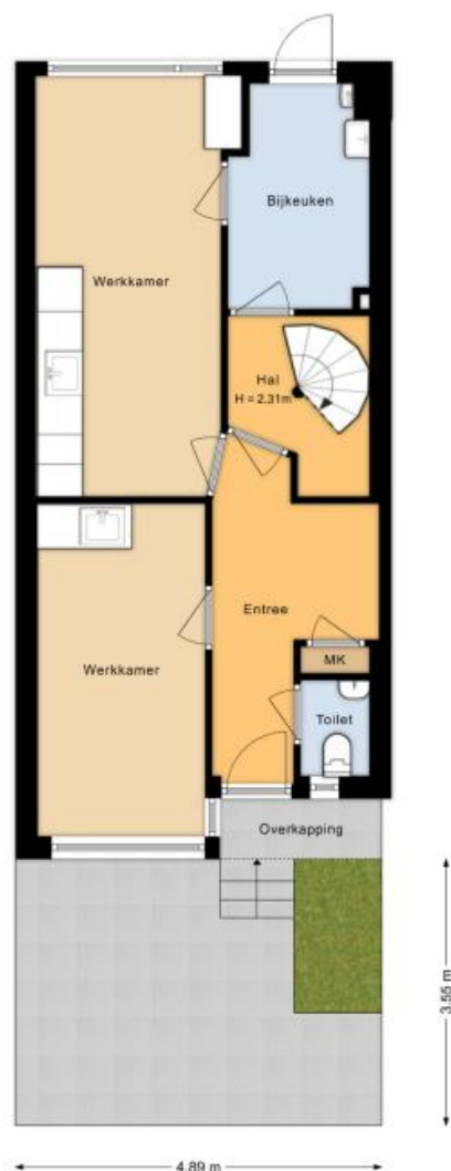
Begane grond Maarten Kruytstraat 6 Noordwijk
