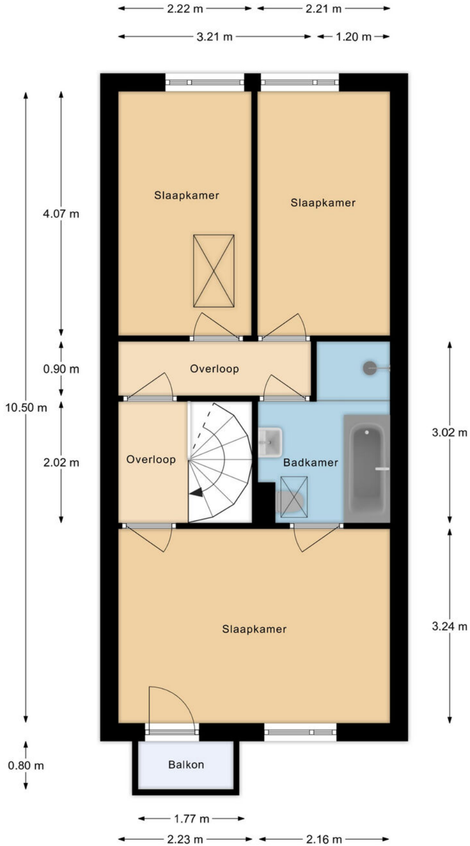
2e Verdieping
