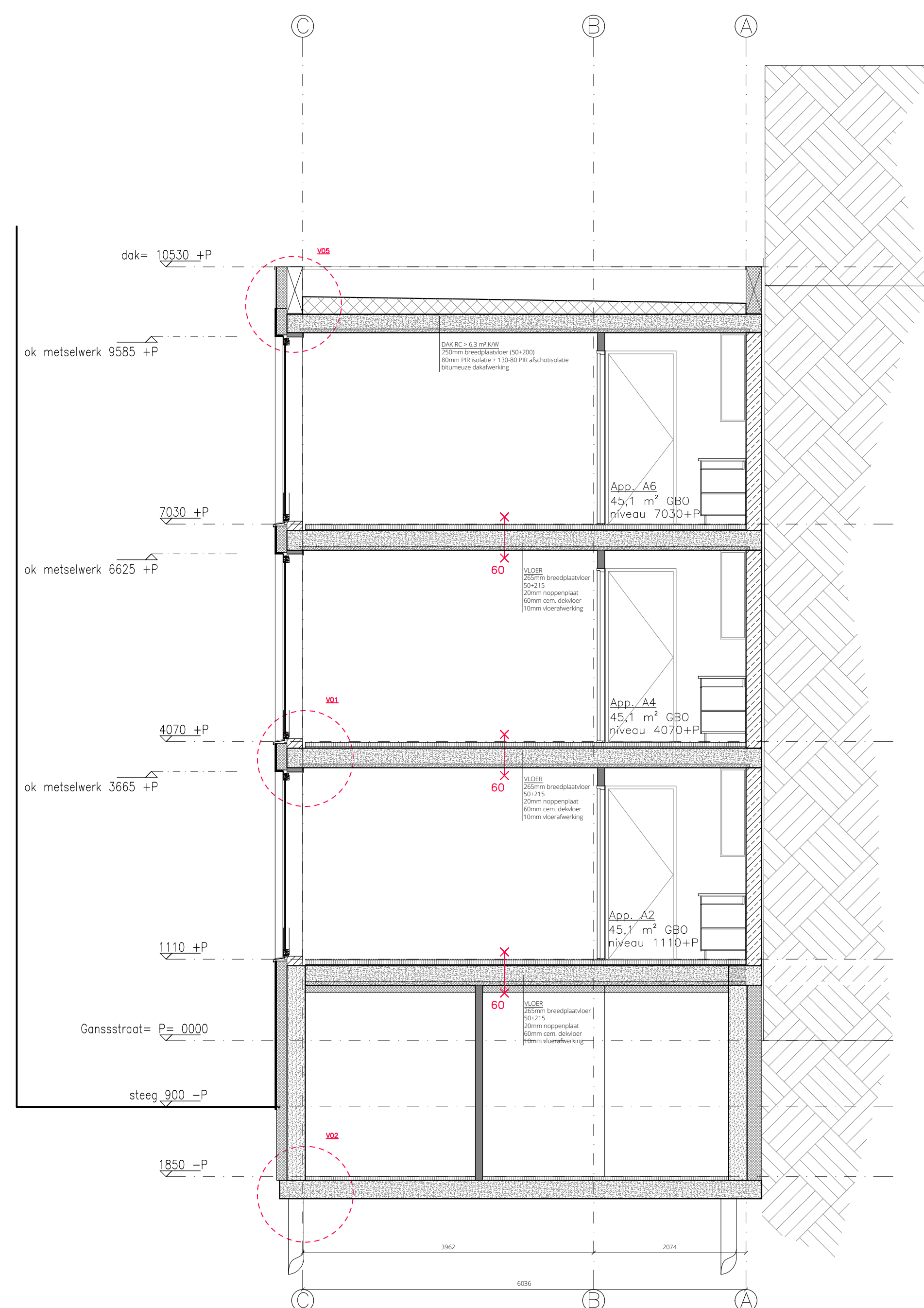
DWARSDOORSNEDE B
