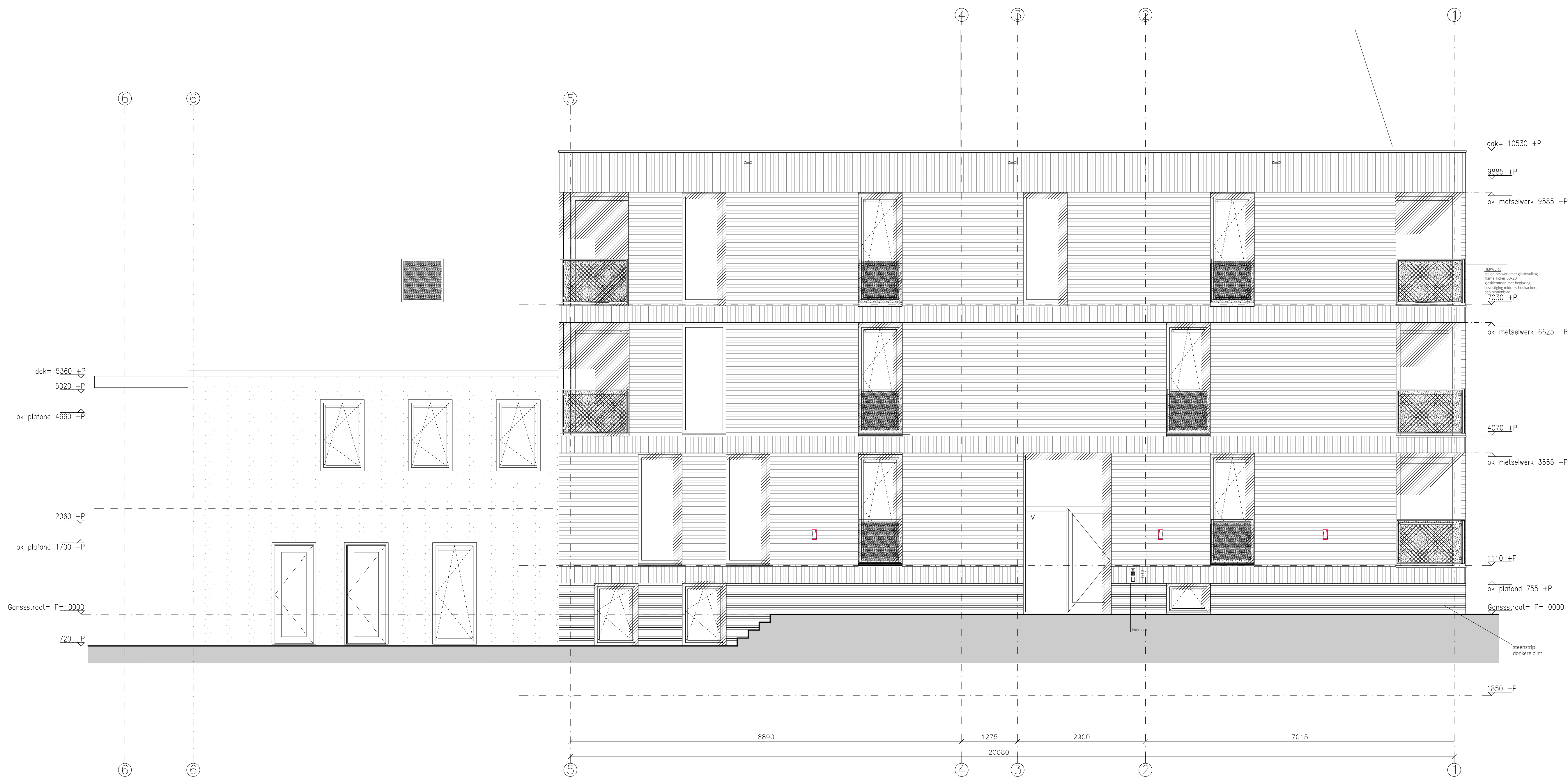
GEVELAANZICHT WESTZIJDE
