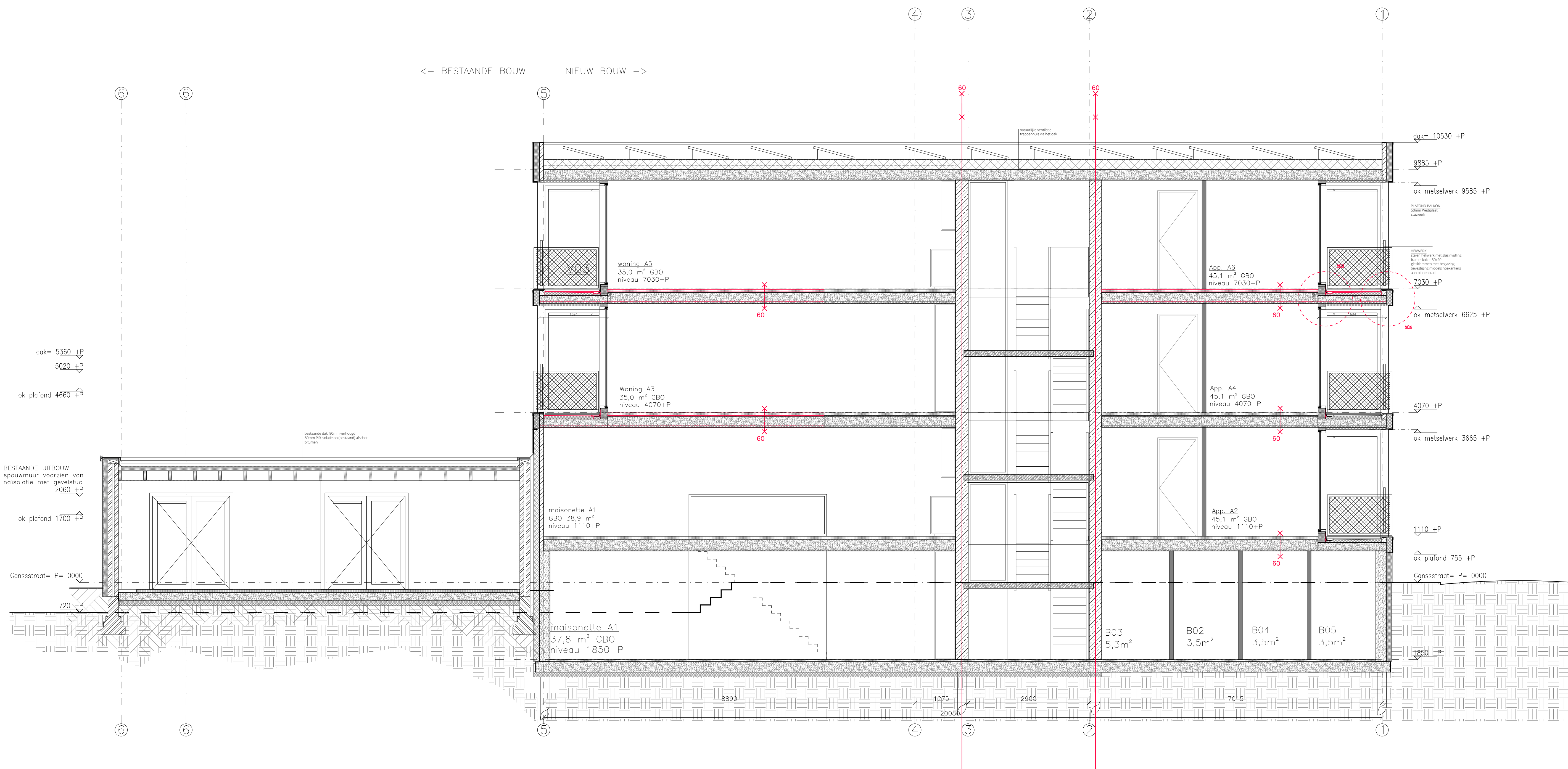
DOORSNEDE A
