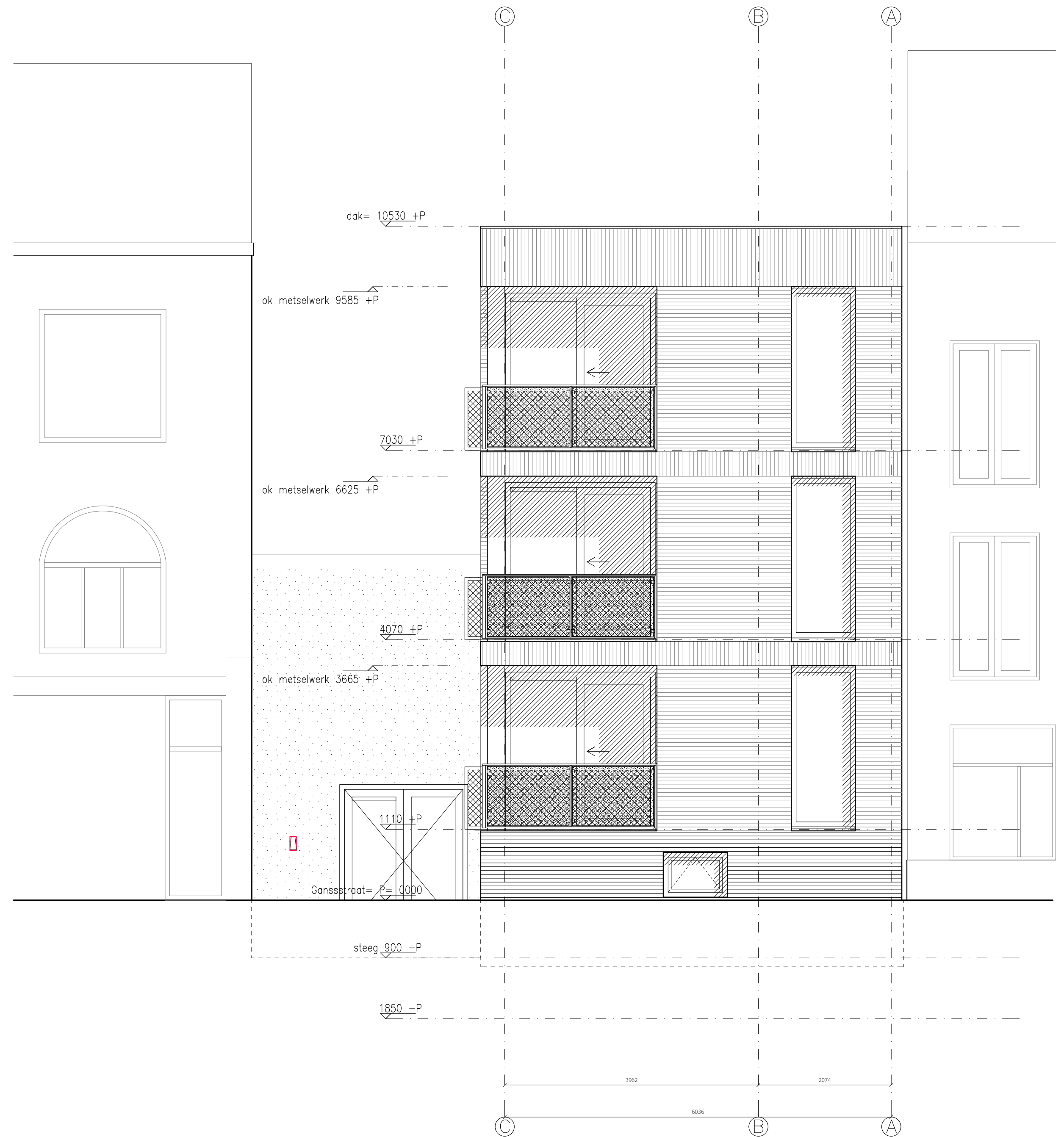
GEVELAANZICHT ZUIDZIJDE
