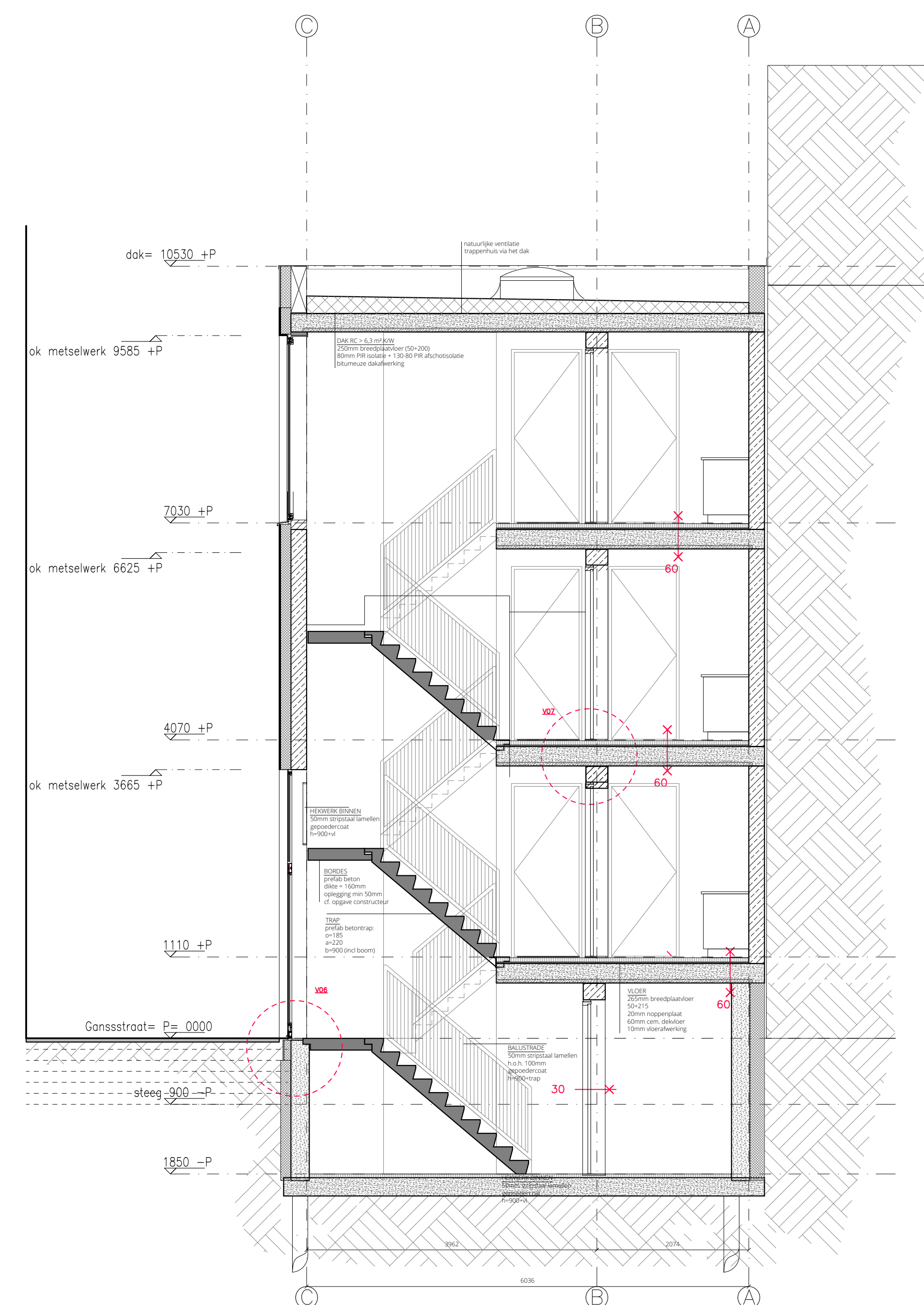
DWARSDOORSNEDE C
