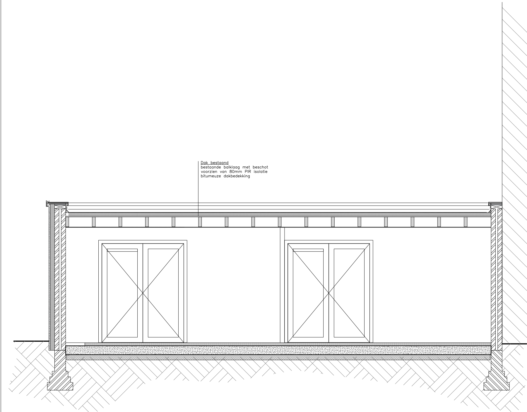
ZUIDOOST GEVEL
