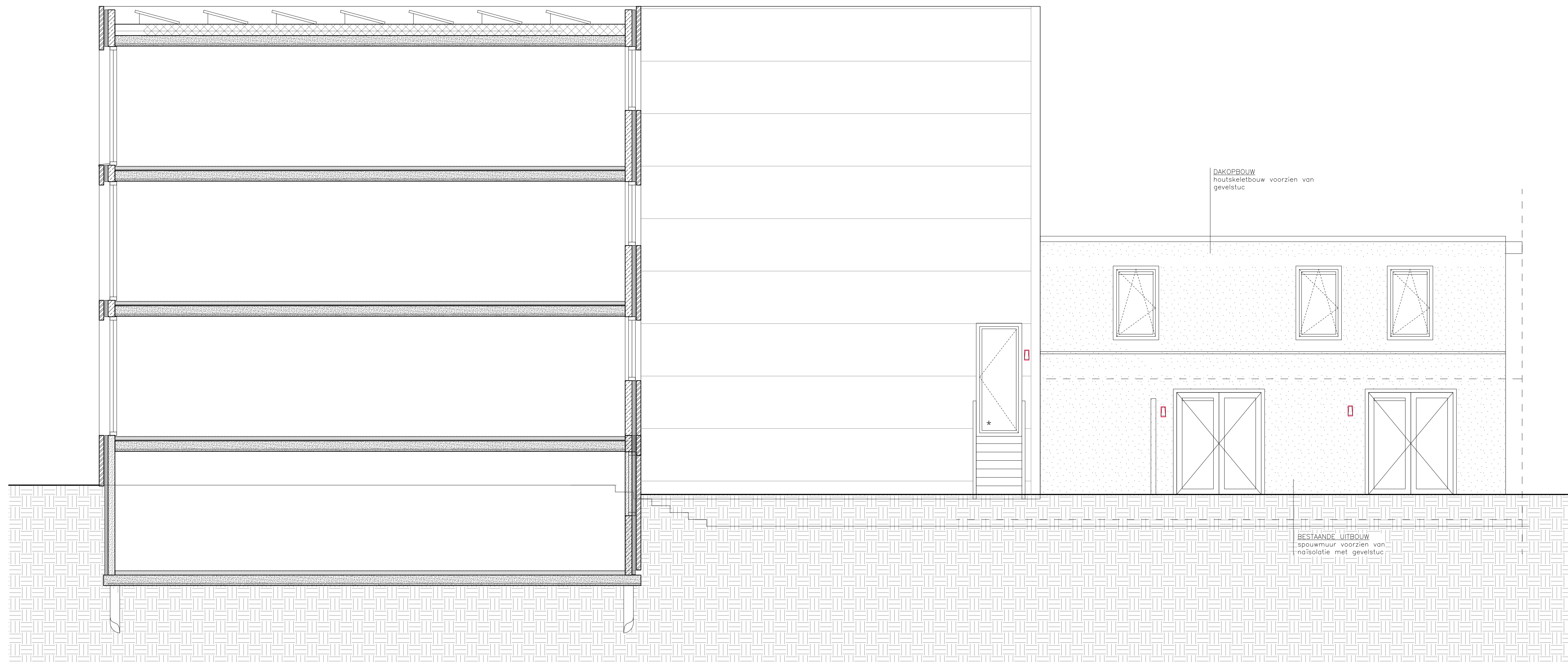
GEVELAANZICHT OOSTZIJDE
