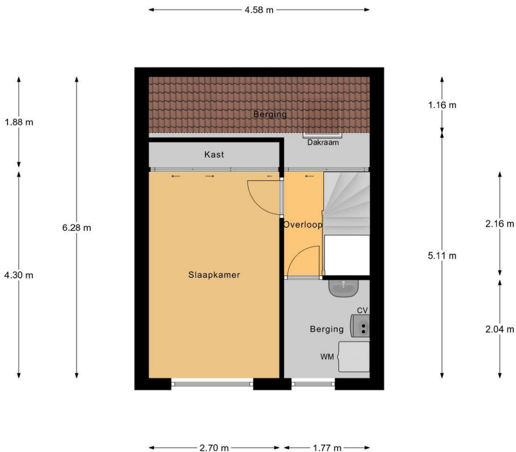
2e Verdieping
