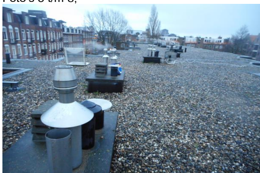
Aanzicht vanaf strang 1 (foto links). Op de foto rechts strang 1 met daarin de enige collectieve afvoerleiding in het complex. Tevens twee kruiskappen aangetroffen (gele pijlen), dit zullen voormalige ventilatie- en verbrandingsluchttoevoerleidingen van de opstellingsruimte (zie ook foto 13 in Bijlage VI).
